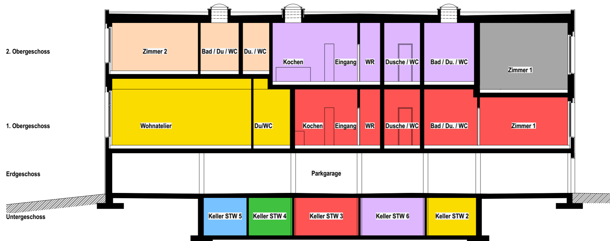
Längsschnitt B-B
